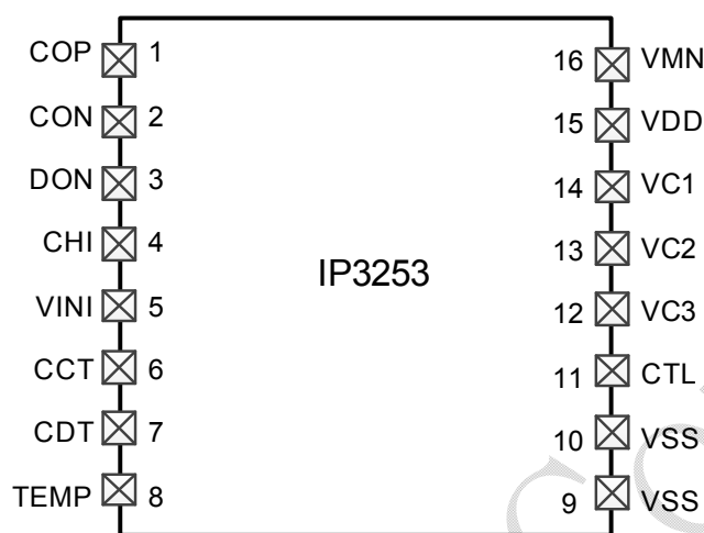
图 1 IP3253 引脚图
